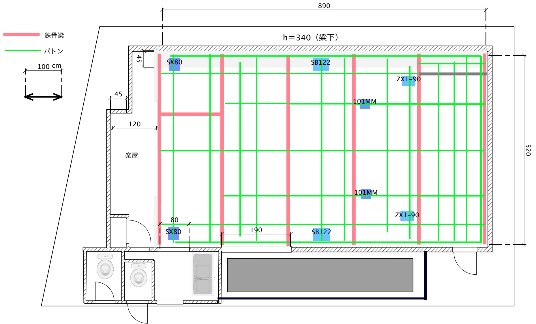
アトリエ第Q藝術 音響SP常設図(1/60縮尺図)
